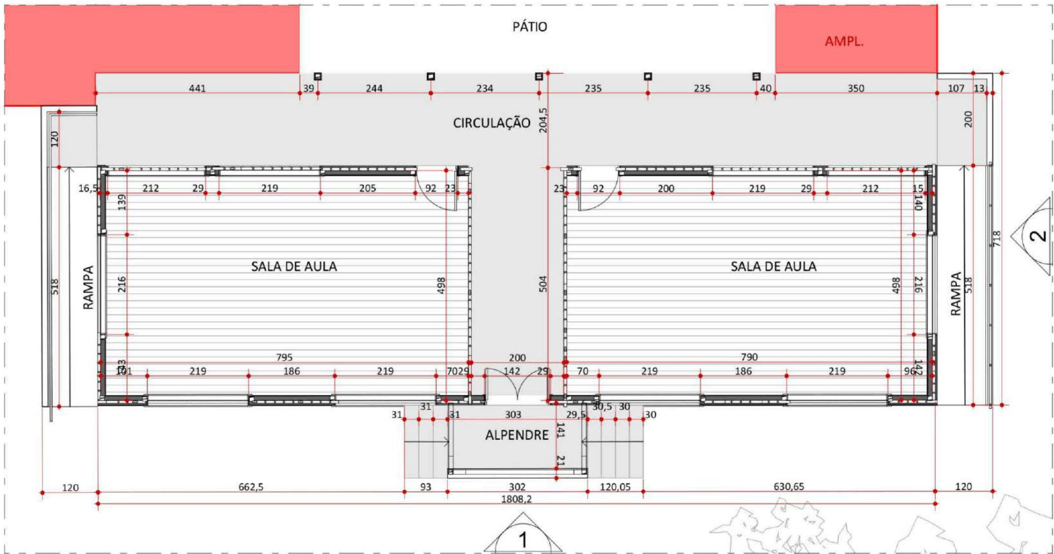
Figura 65 - Planta da Escola Municipal Padre Anchieta.
