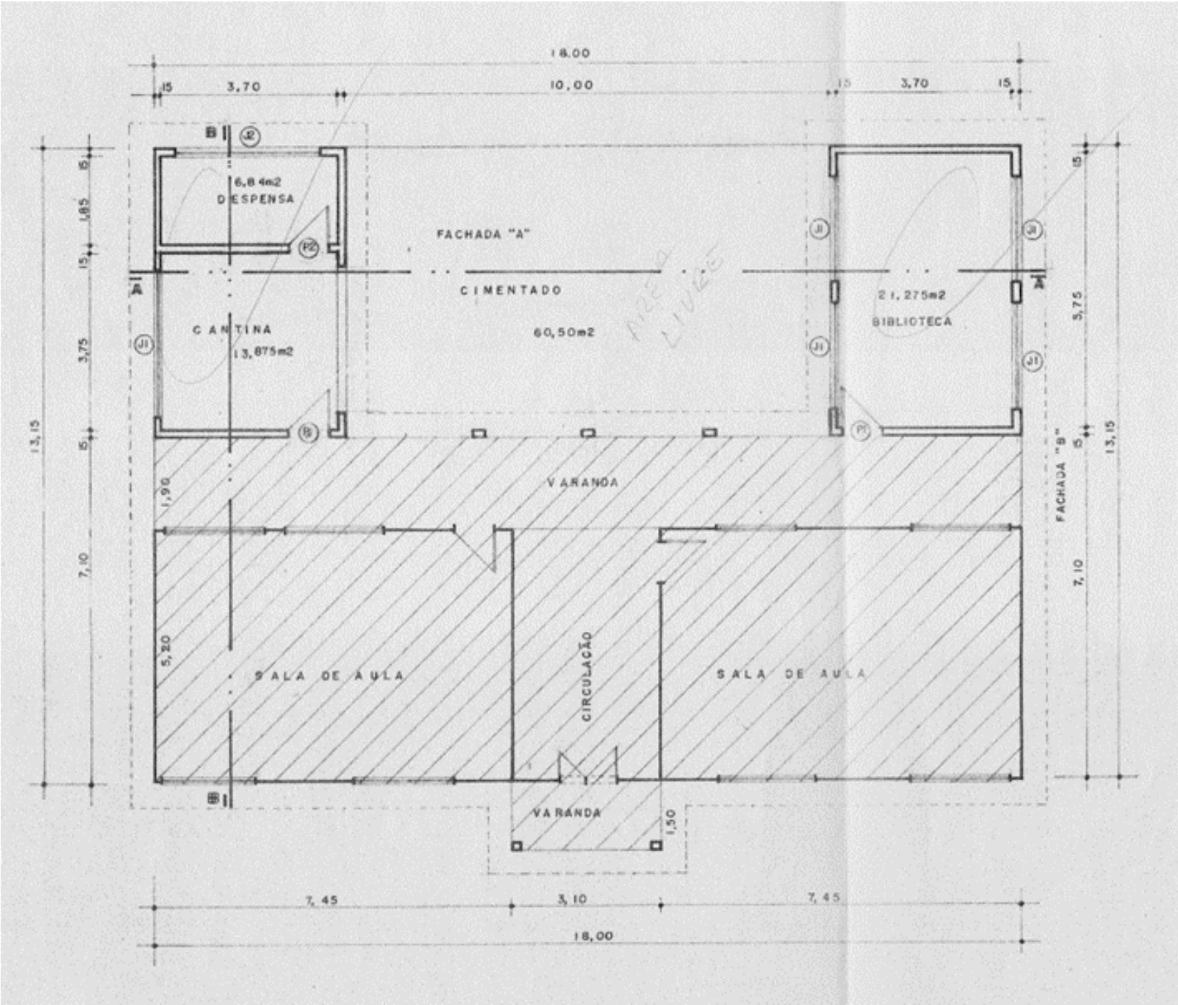
Figura 69 - Planta Baixa da Escola antiga com anexos.
