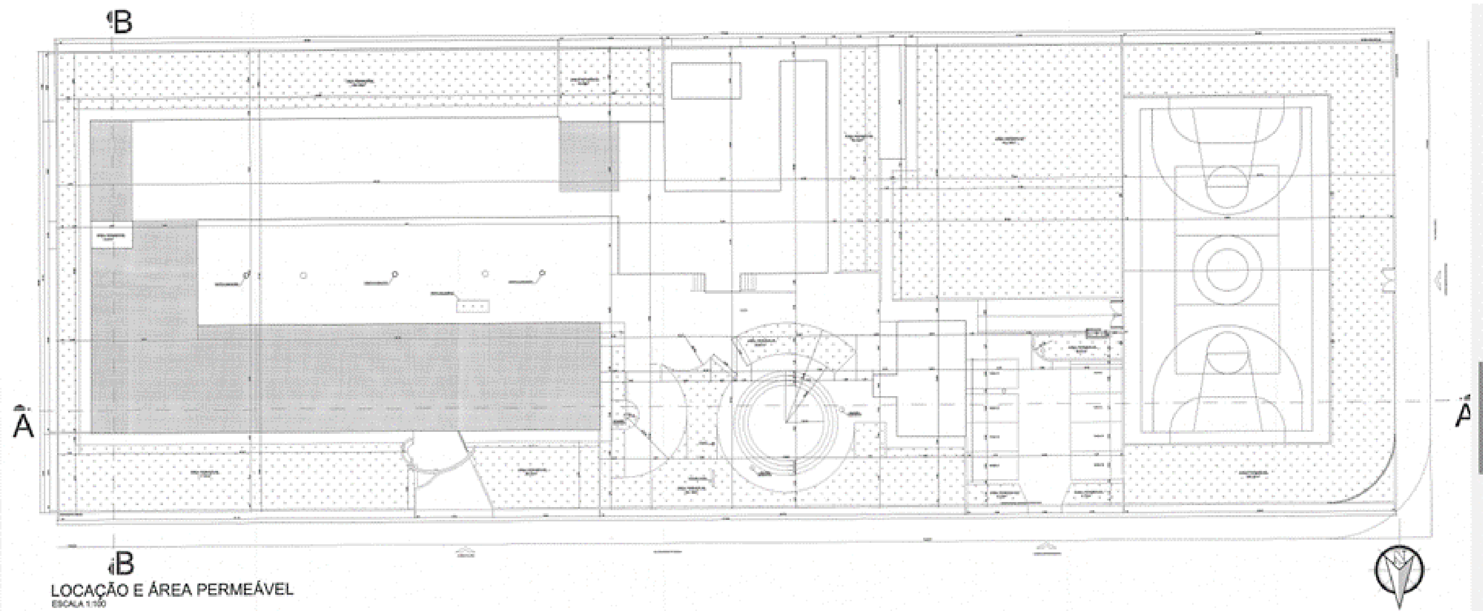
Figura 71 - Projeto arquitetônico aprovado em 2002.
