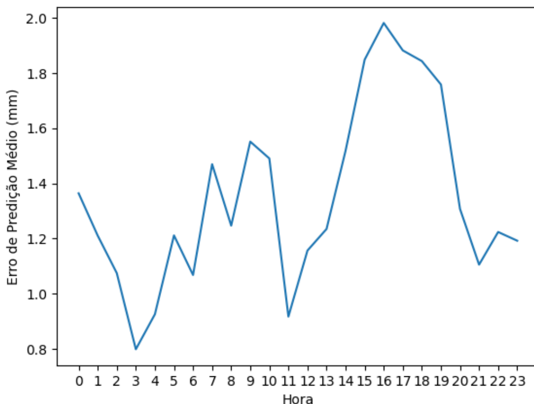
Figura 11 – Média de erros por hora
