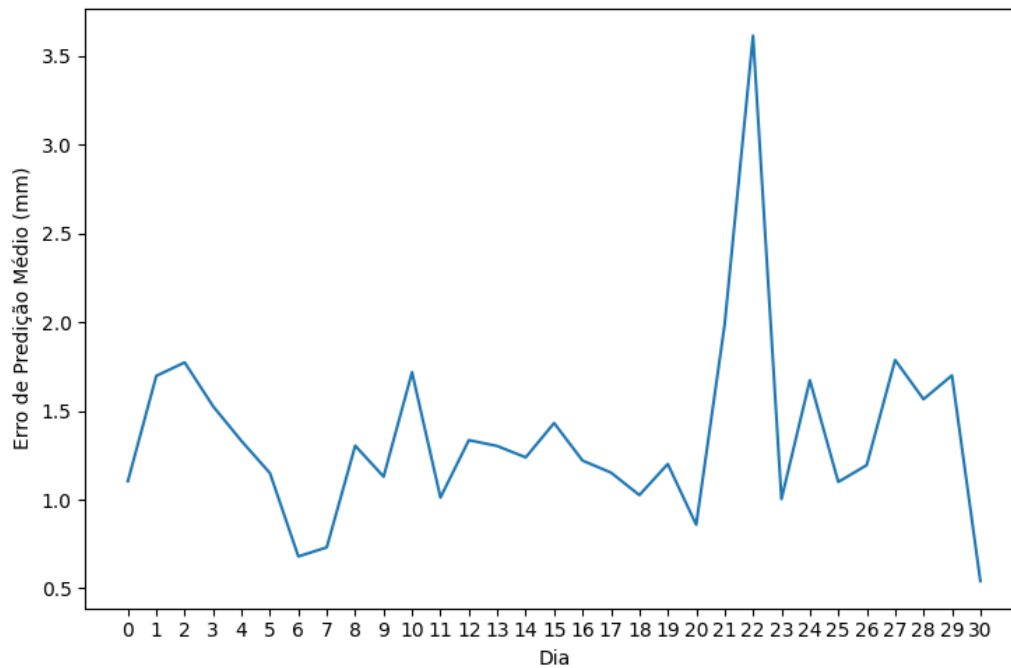
Figura 12 – Média de erros por dia
